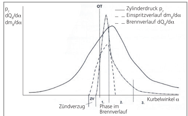
Bild 1: Die drei Phasen des Verbrennungsablaufs Quelle: Handbuch Schiffsbetriebstechnik, Seehafen Verlag
